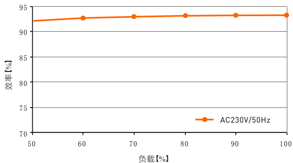
效率与负载关系图
